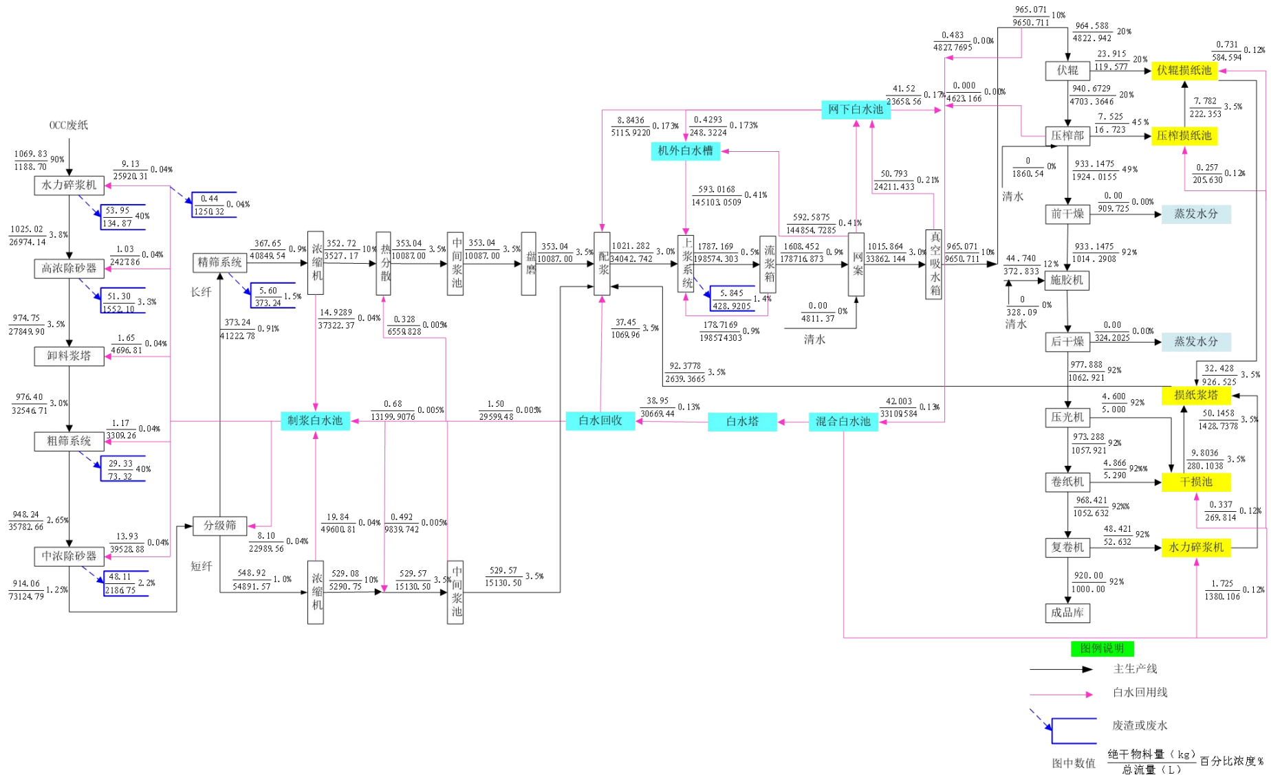
图 4-9 瓦楞原纸生产线浆水平衡图
