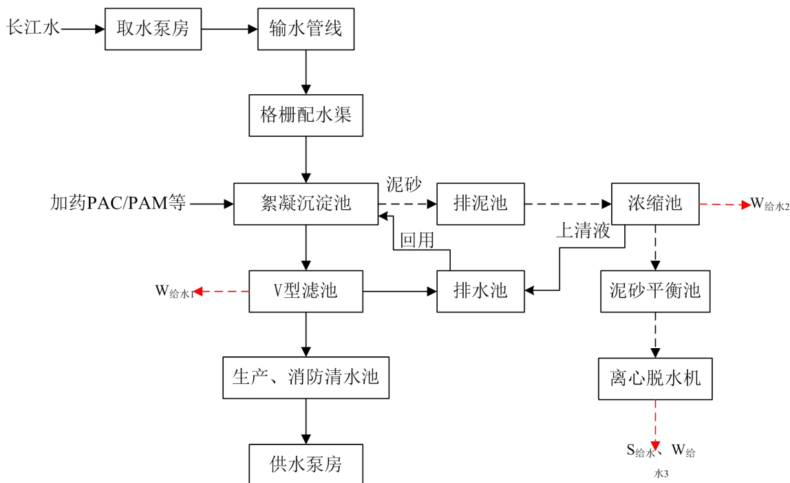
图 4-5 给水站工艺流程及产污节点图
