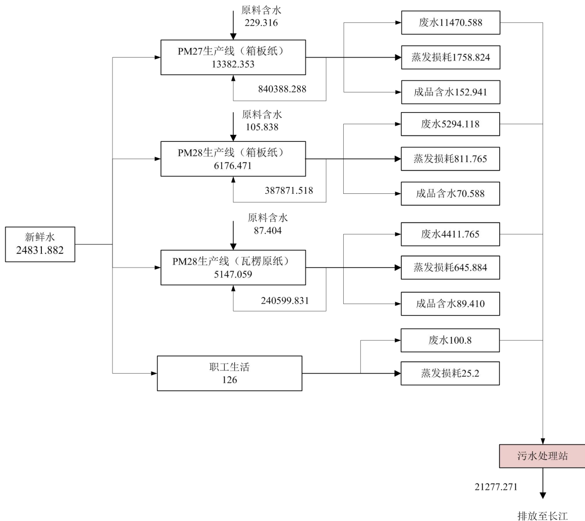
图 4-10 本项目水平衡示意图（单位：m³/d）
