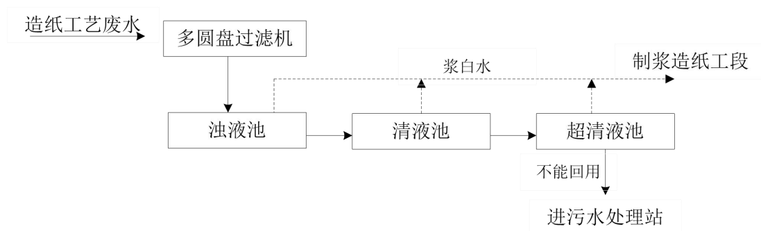
图 8-1 项目白水回收系统工艺流程示意图
