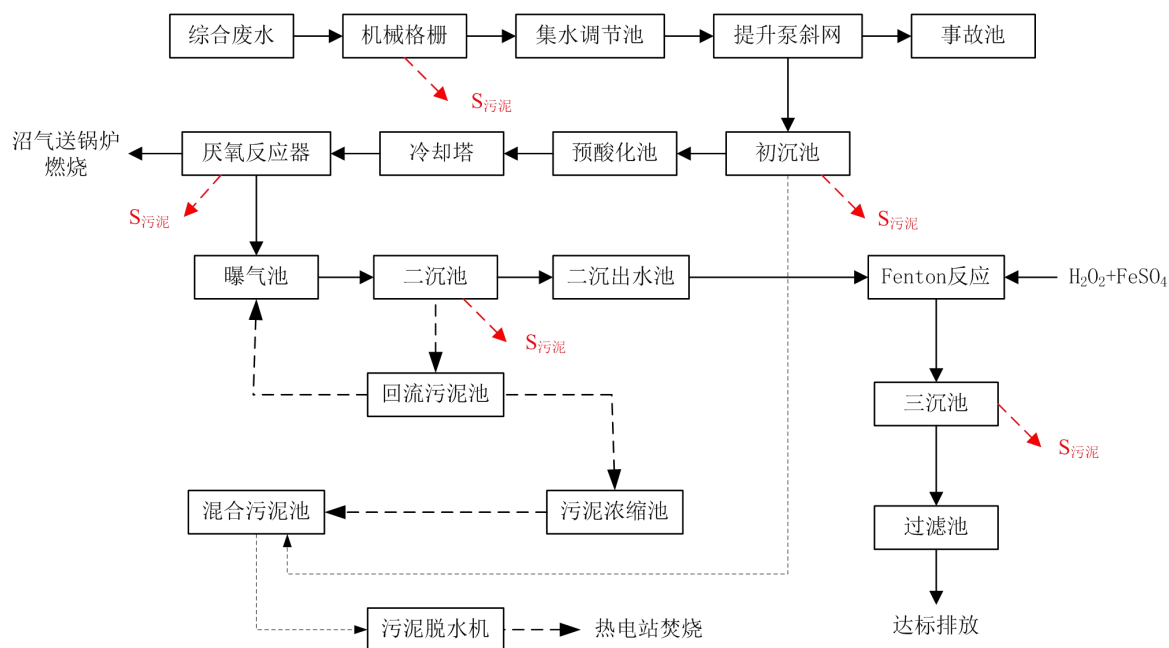
图 4-6 污水处理站工艺流程和产污节点
