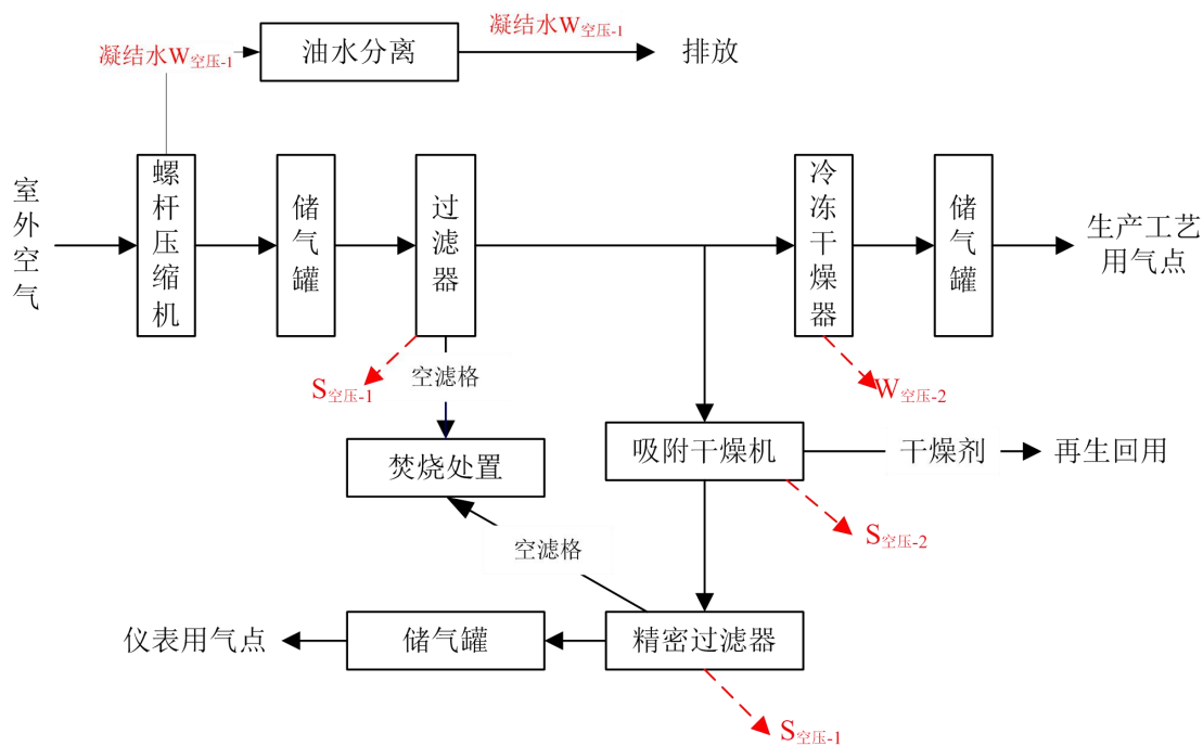
图 4-7 空气压缩站工艺流程及产污节点分析示意图
