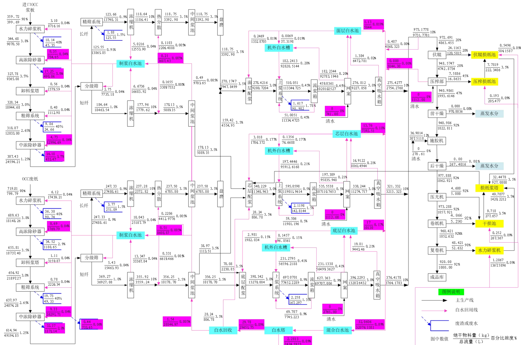
图 4-8 箱板纸生产线浆水平衡图
